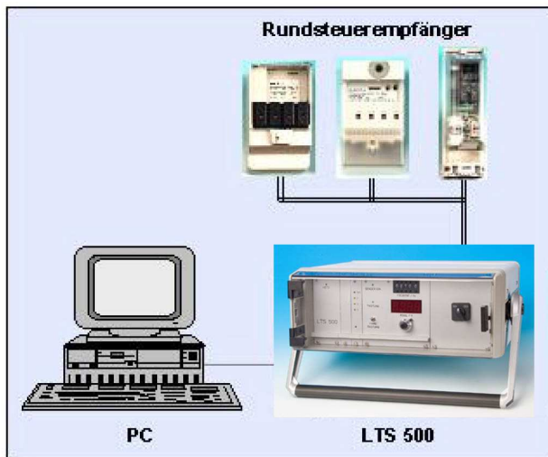
Prinzipieller Aufbau des Empfängerprüfplatzes
